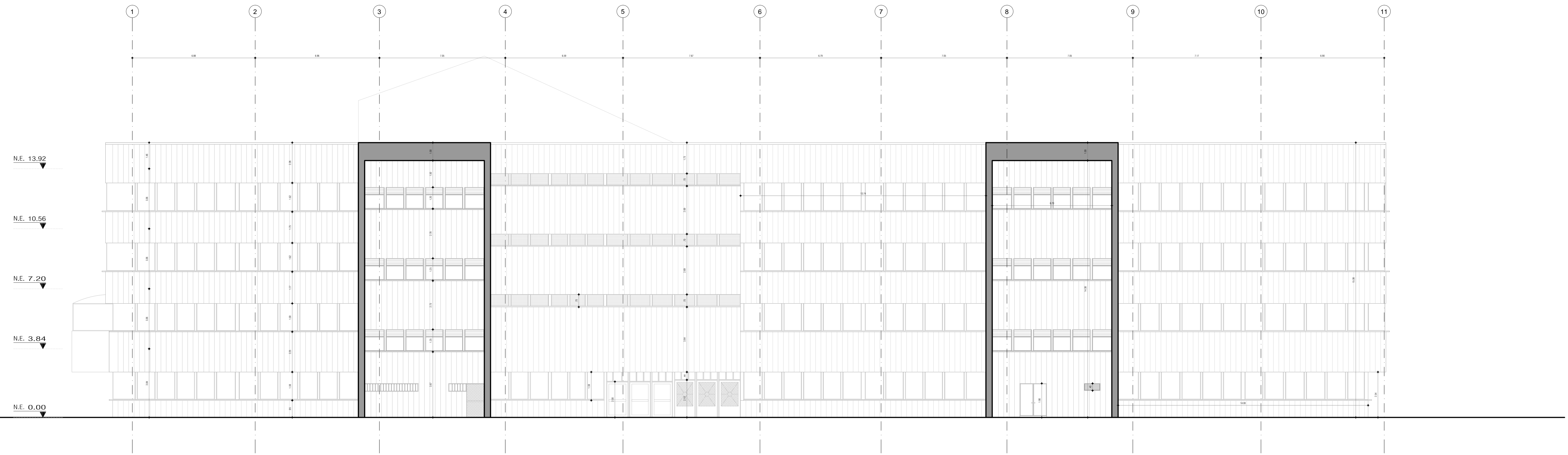
A-201 EDIFICIO-B FACHADA FRONTAL ESC 1:75
